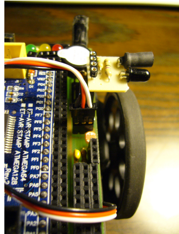
PWM Dret
